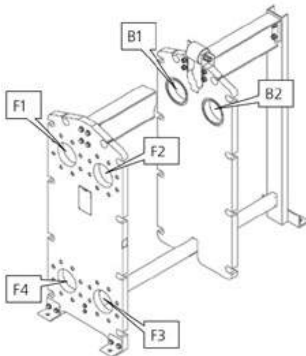
Рис. 2 - Верхнее расположение
